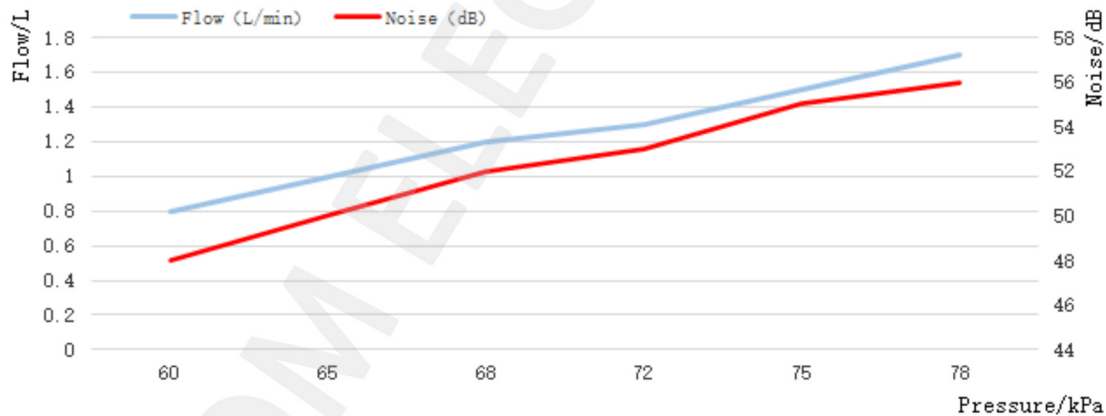
特性曲线图 Characteristic curve: 流量和噪音变化
